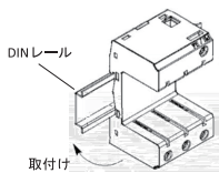
DIN レールへの取付け
