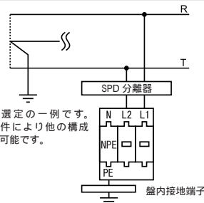
4. 三相 3 線 結線 AC200V 接地線あり
